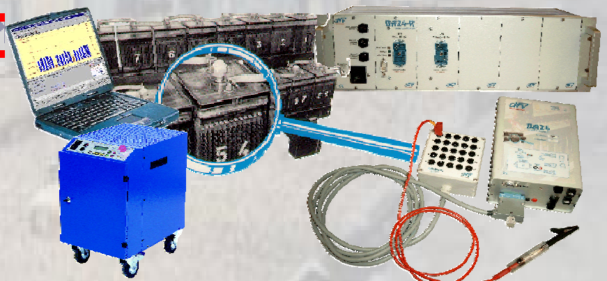
Testeurs automatiques de batteries BATCAT et bancs de décharge
